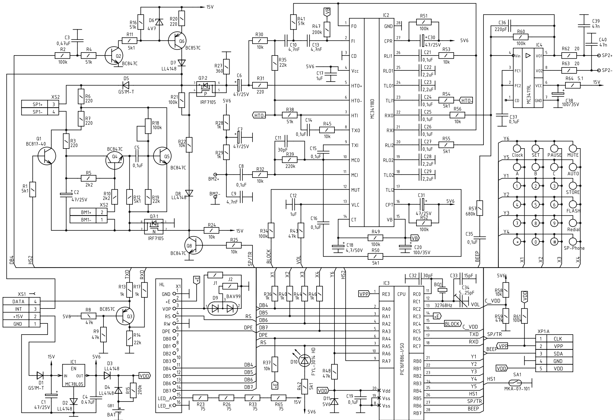
Модуль управления ТК401DN Схема электрическая принципиальная
