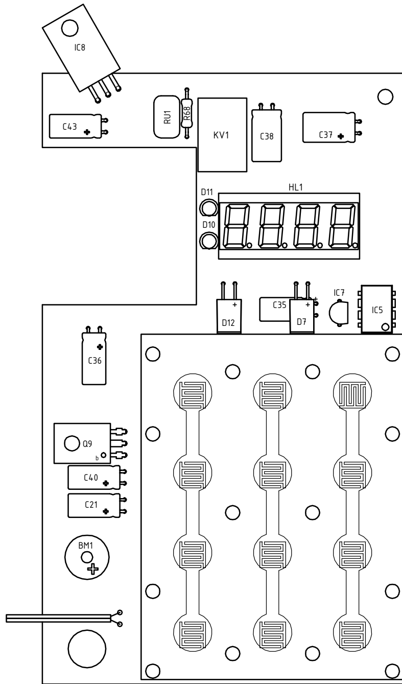
Плата БВД-СМ101РСРЛ Сборочный чертёж
