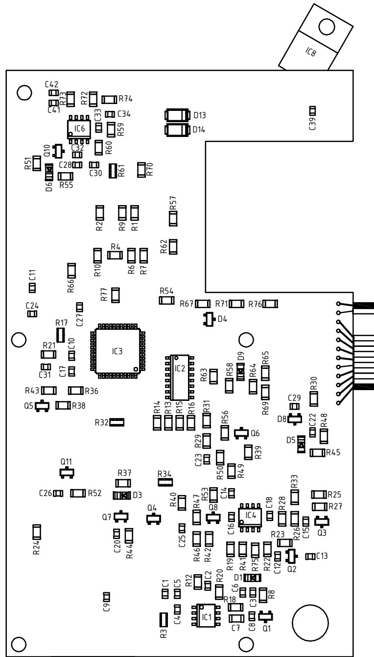
Плата БВД-СМ101РСРЛ Сборочный чертёж
