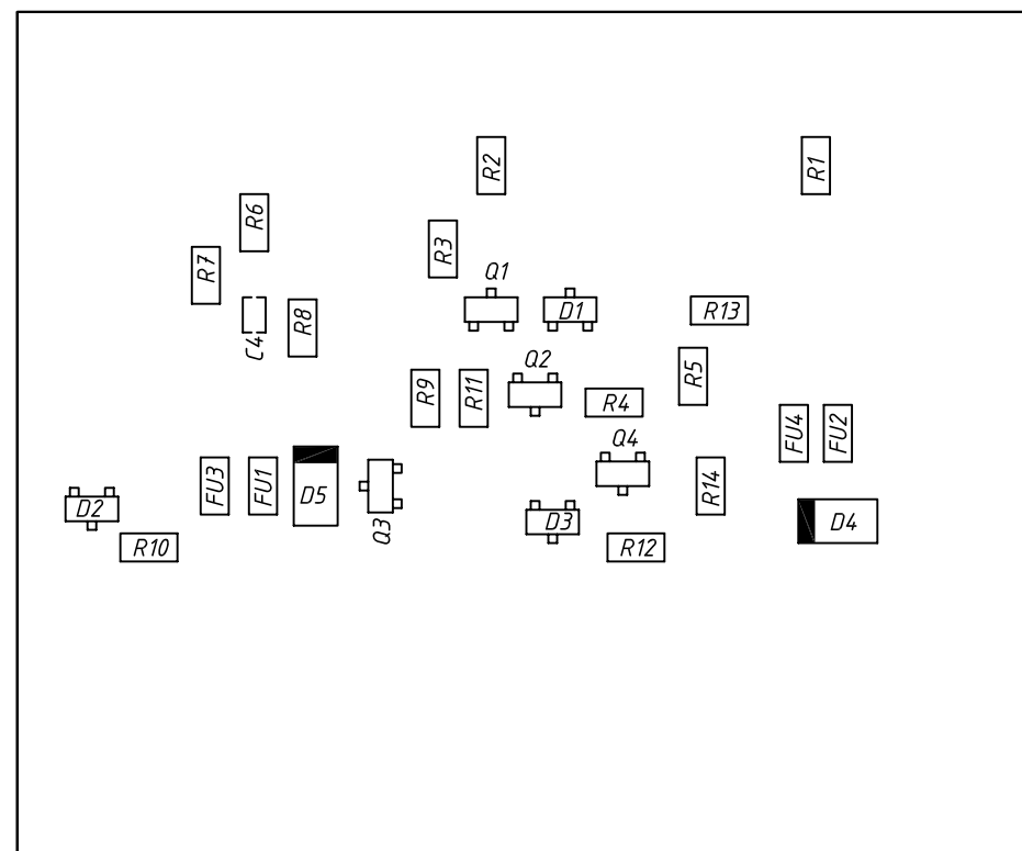
Плата РВС-2 Сборочный чертеж
