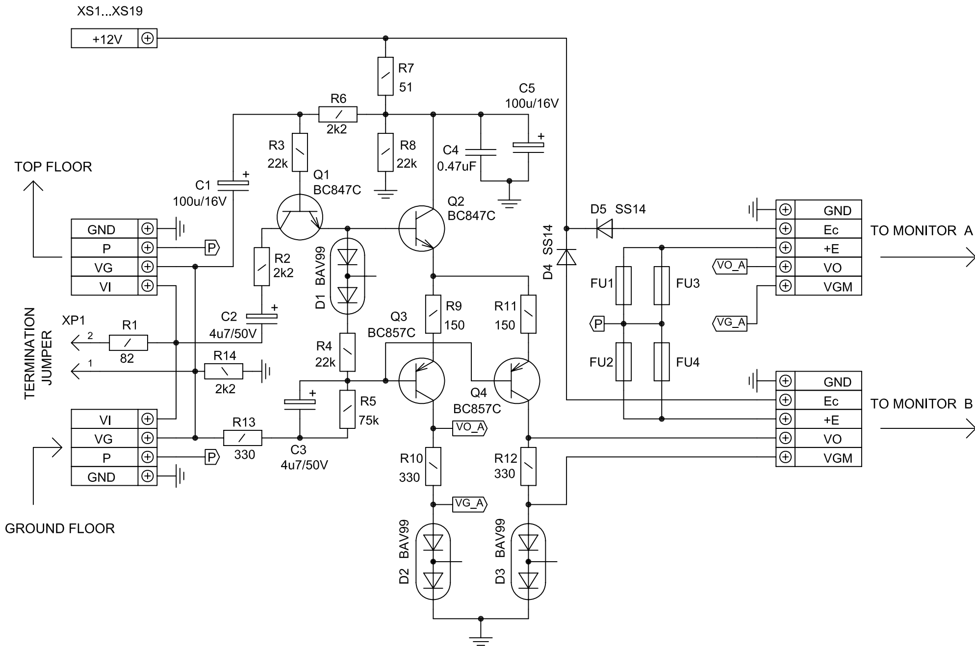
Разветвитель видеосигнала PBC-2 Схема электрическая принципиальная
