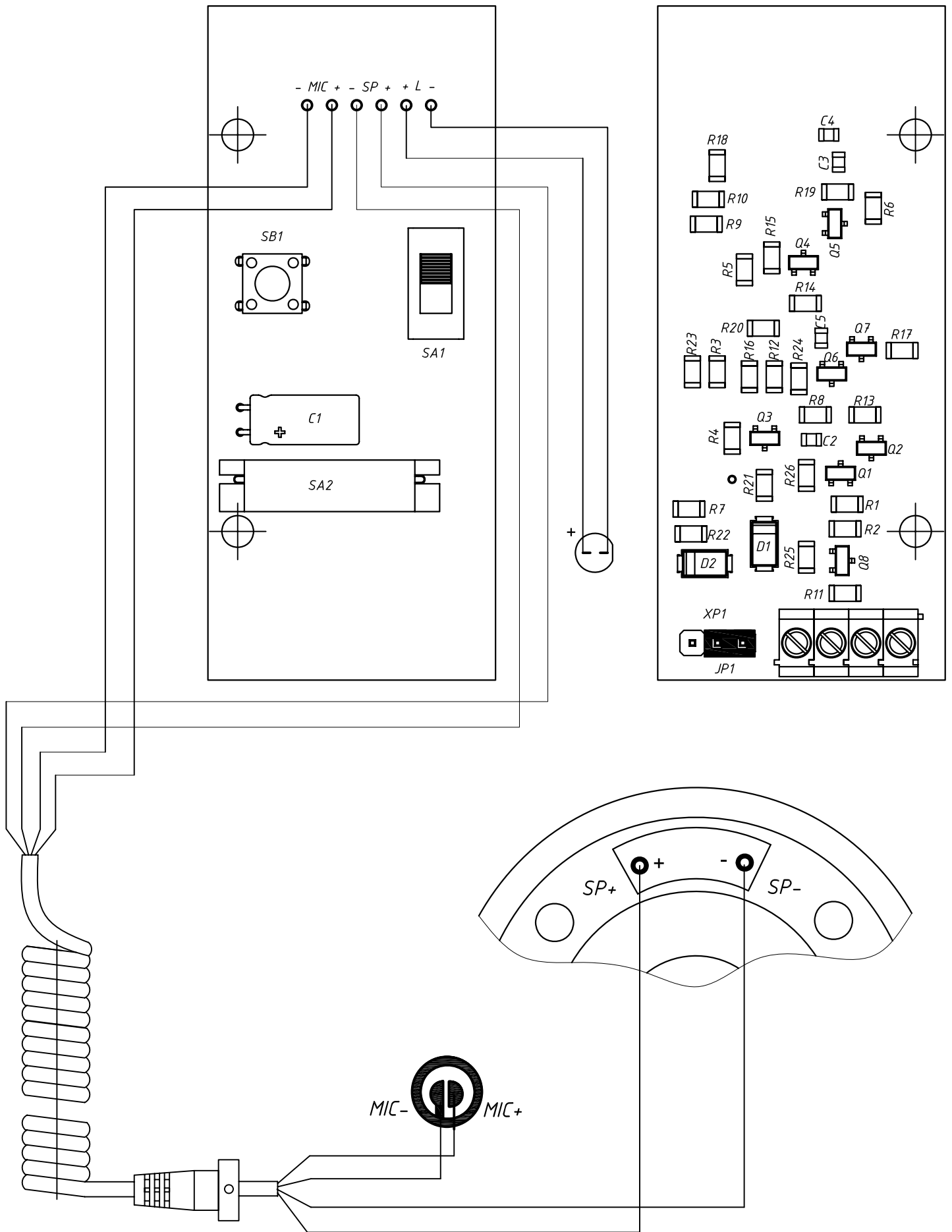
Плата УКП-12-1 Сборочный чертеж
