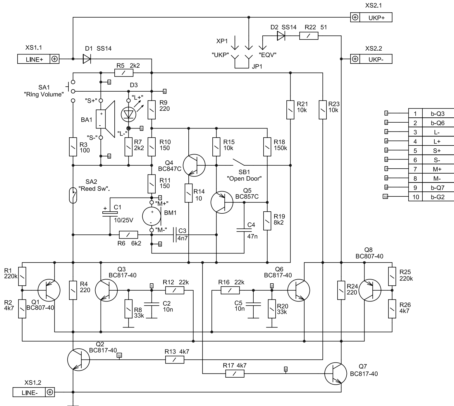
Устройство квартирное переговорное УКП-12-1 Схема электрическая принципиальная
